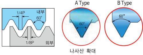
나사산 확대
